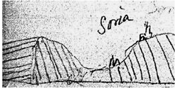
6. Dibuix de Charles Lyell de 1830 on es veu la falla de Mig-Món (Cortesia de Lord Lyell de Kinnorby).
