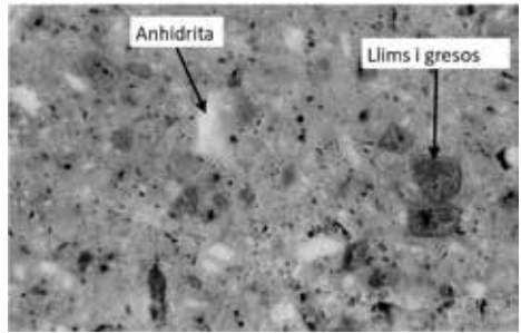
Figura 7: Imatge al microscopi del morter de guix analitzat.
